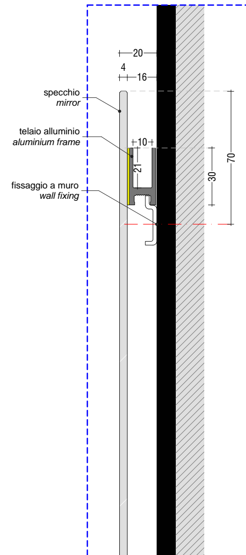
DETTAGLIO SISTEMA DI AGGANCIO SPECCHIO DETAIL_SUPPORT MIRROR
