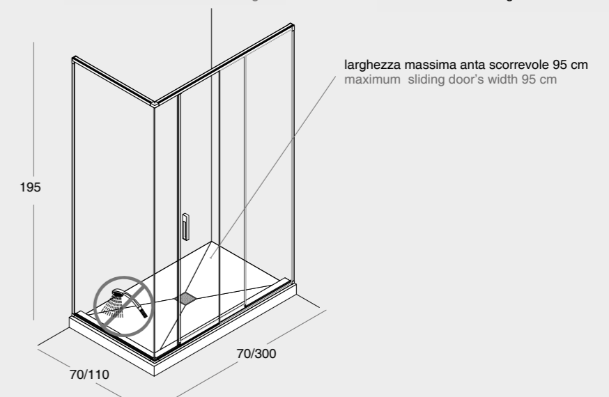
anta laterale / lateral sliding door
