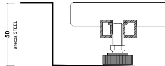
PIEDINO REGOLABILE / adjustable feet
